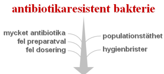
Figur 2 Schematisk beskrivning av faktorer som bidrar till spridning av antibiotikaresistenta bakterier.
